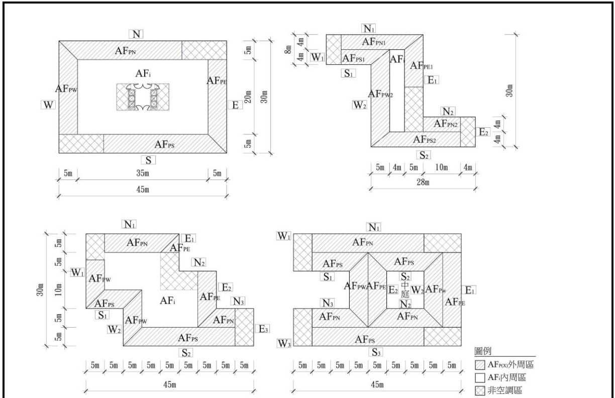
圖 3 建築物外周區範圍（外牆中心線起算深度 5m 內）
